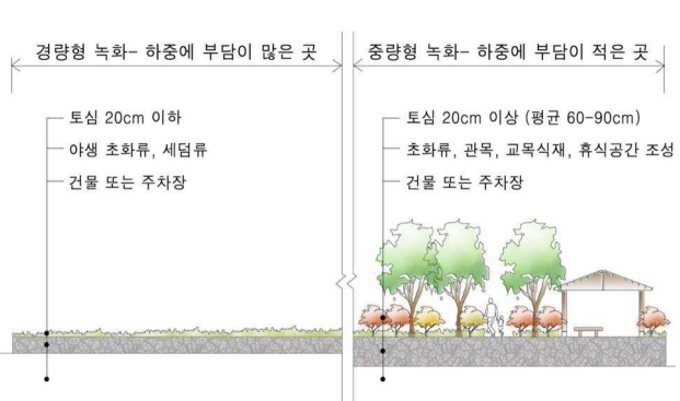
[그림4-6-2] 인공지반 활용 예시도
