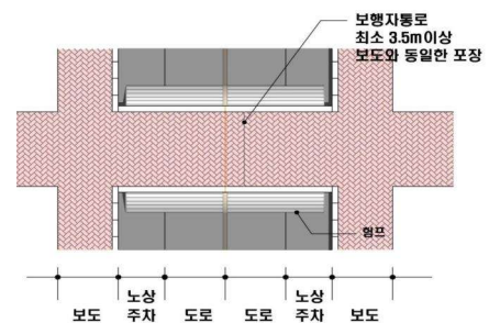
[그림 1-1-13] 보행자우선구조 예시도
