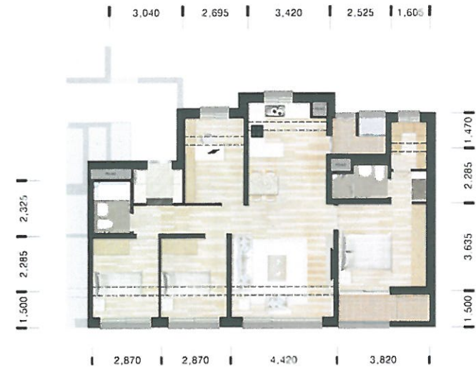
74B 단위세대 평면도(확장형)
